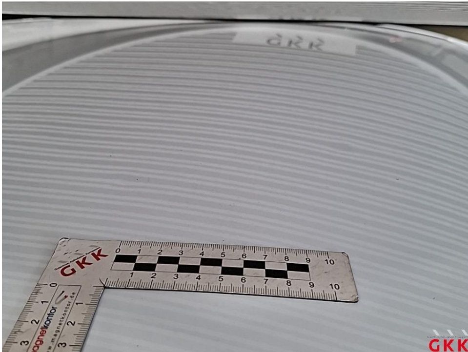
Bild 48. Dach, 4 bis 10 Dellen / Bauteil, kalt drücken
