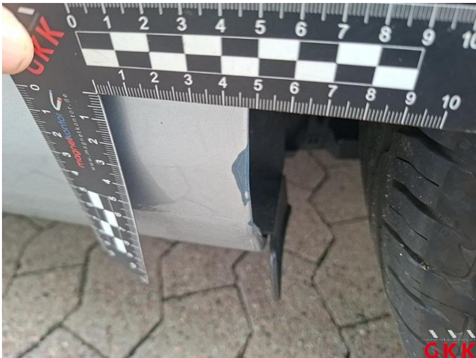
Bild 44. Seitenwand links, Reparaturmangel, instand setzen - lackieren
