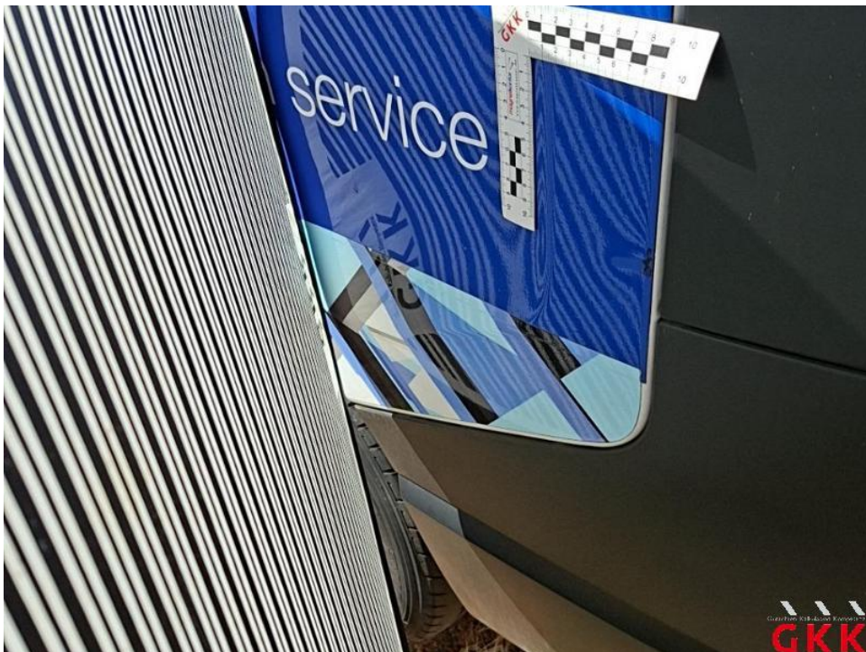
Bild 76. Seitenwand links, bis 3 Dellen / Bauteil, kalt drücken
