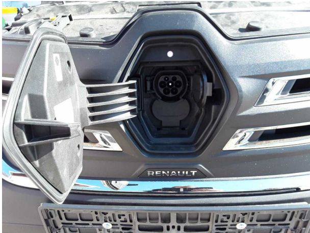
Abbildung 13: Ladebuchse/Tankstutzen
