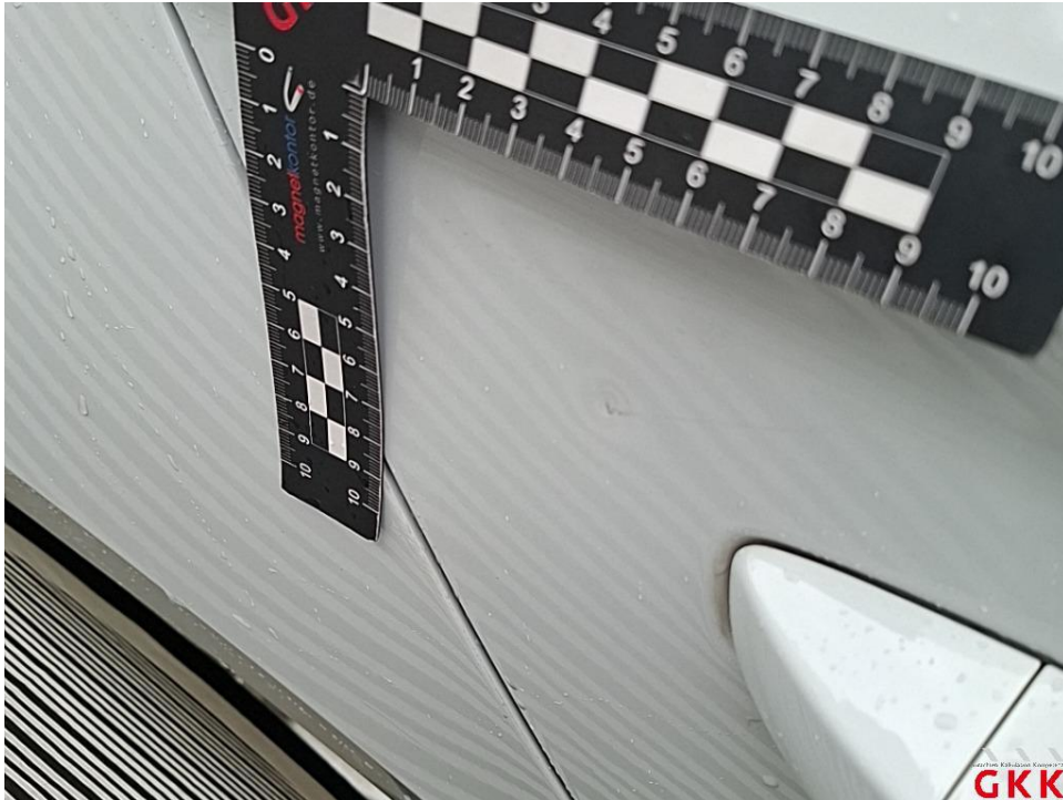
Bild 15. Tür hinten rechts, bis 3 Dellen / Bauteil, Smartrepair
