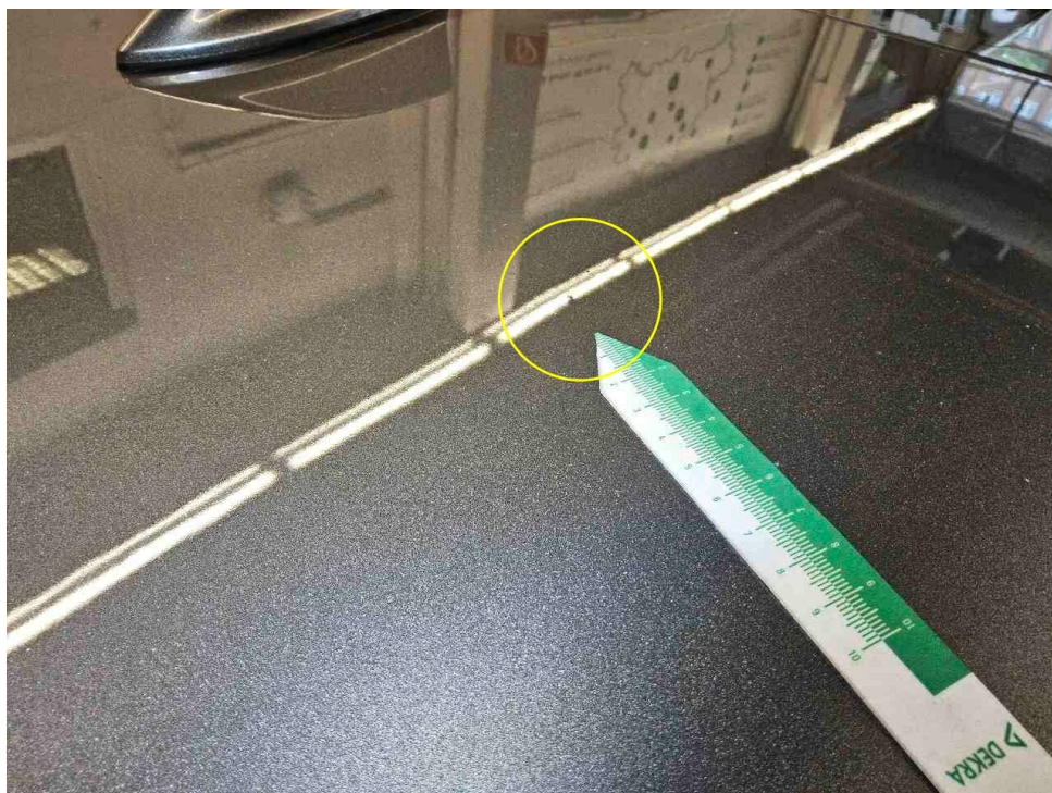
Bild 18 : Ringsum instandgesetzt/nachlackiert außer Dachholm links und rechts, nicht sach- und fachgerecht instandgesetzt/ nachlackiert
