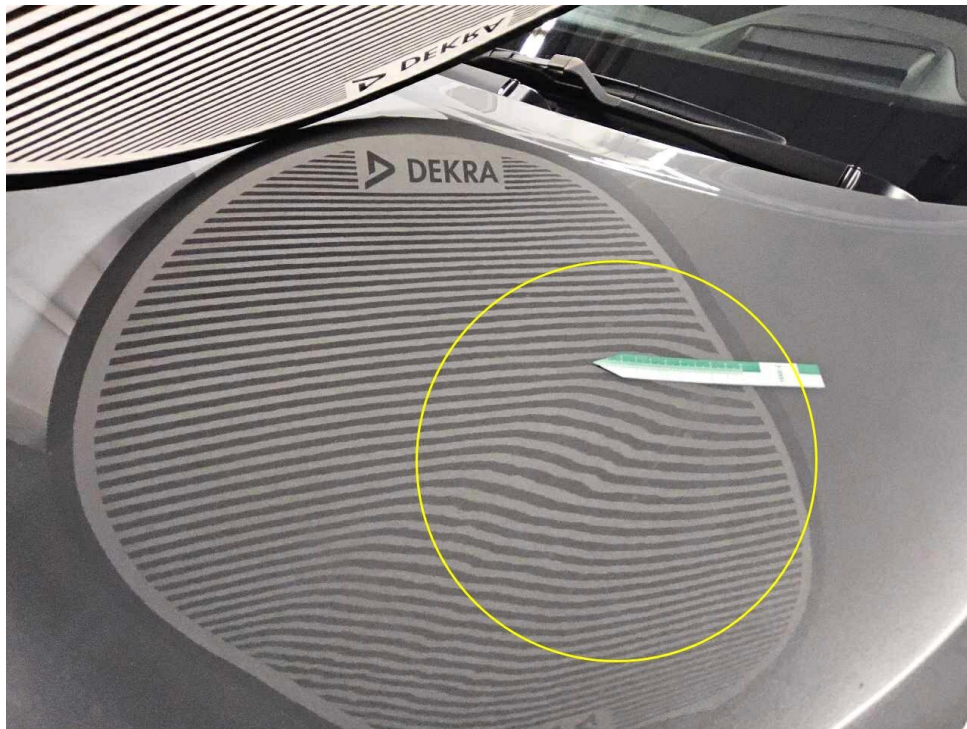
Bild 17 : Ringsum instandgesetzt/nachlackiert außer Dachholm links und rechts, nicht sach- und fachgerecht instandgesetzt/ nachlackiert
