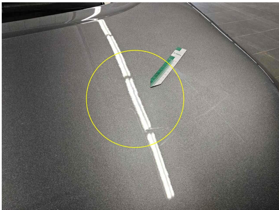
Bild 16 : Ringsum instandgesetzt/nachlackiert außer Dachholm links und rechts, nicht sach- und fachgerecht instandgesetzt/ nachlackiert
