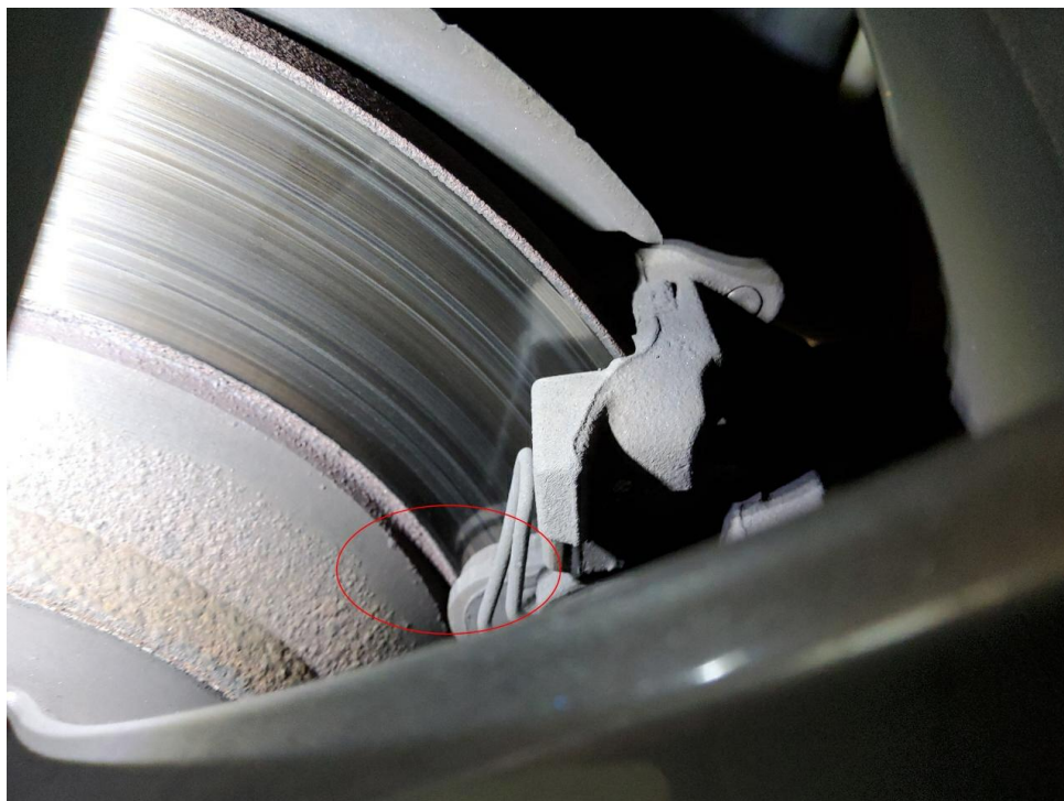
Bild 24 : Bremse hinten, Bremsbeläge und Bremsscheiben, Verschleißgrenze erreicht
