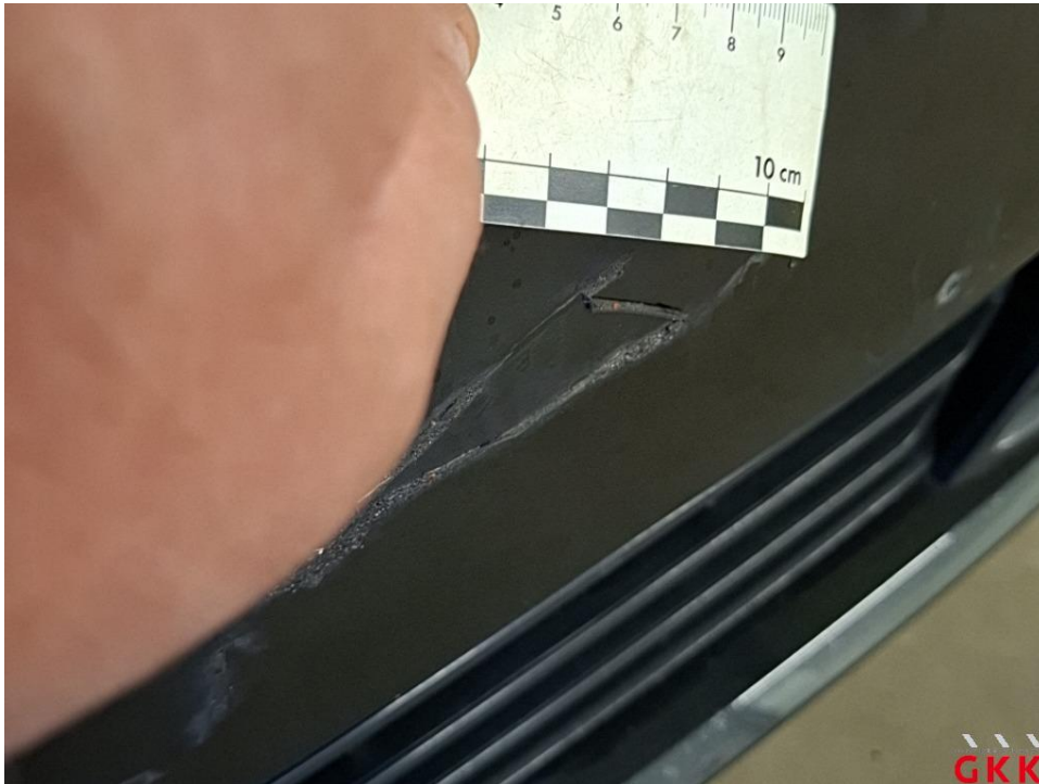
Bild 19 Stoßfänger vorne, Verkleidung -lackiert-, gerissen, ersetzen
