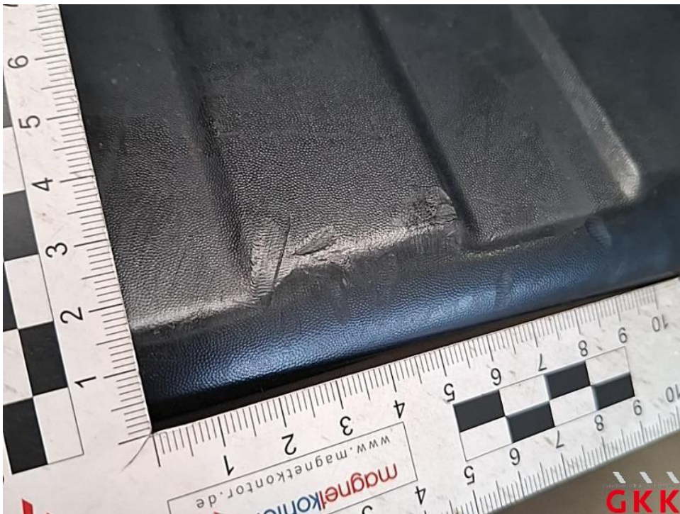
Bild 42. Stoßfänger hinten, Verkleidung -unlackiert-, beschädigt, ersetzen
