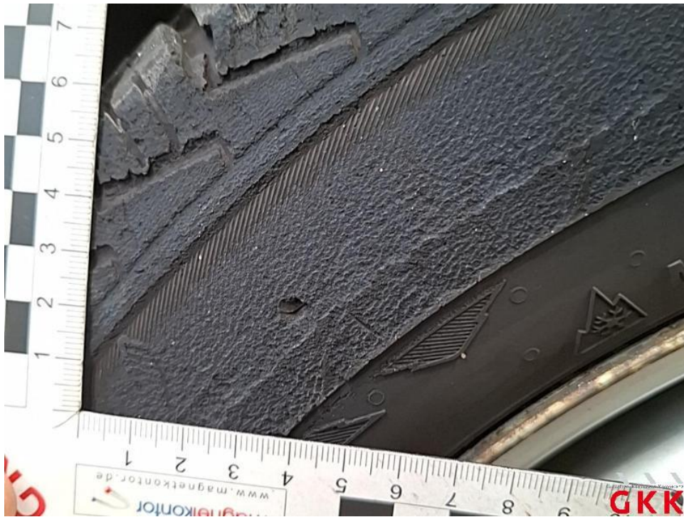
Bild 23. Reifen, vorne rechts, beschädigt und Untermaß, ersetzen
