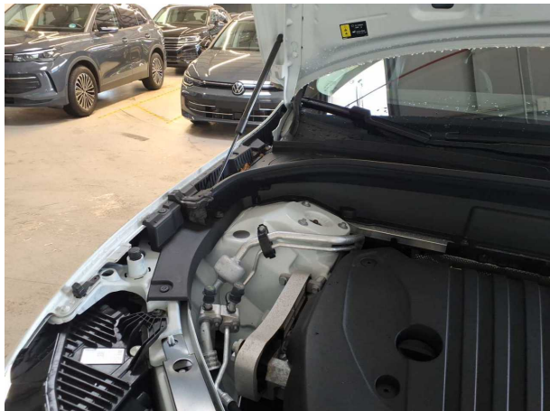
Beschädigung #1: Kotflügel rechts: Kotflügel rechts (Dämmung) - Marderschaden - erneuern
