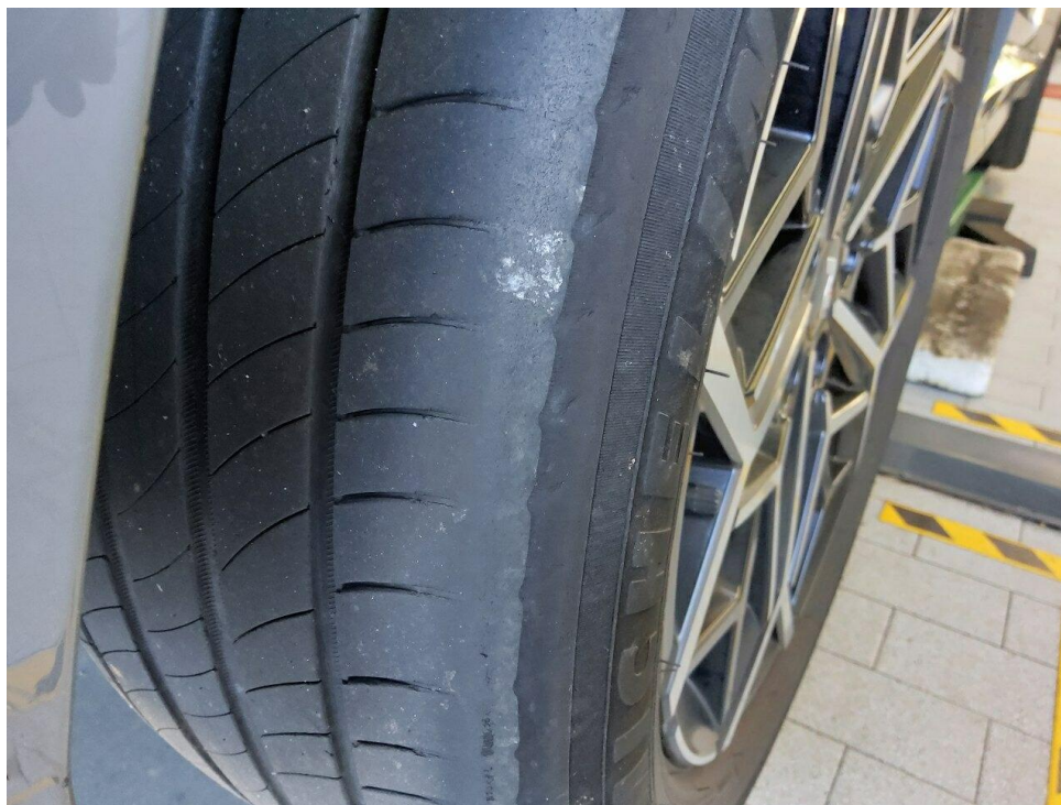
Bild 8 : Reifen hinten rechts aussen abgelaufen
