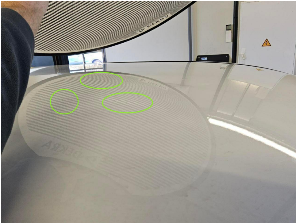
Bild 11 : Dach, Restspuren aus Instandsetzung, noch Dellen vorhanden
