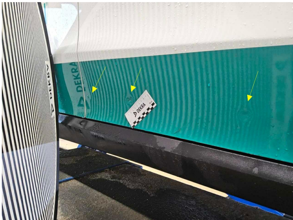
Bild 18 : Tür vorne rechts, deformiert, instandsetzen und lackieren mit Lackaufbau
