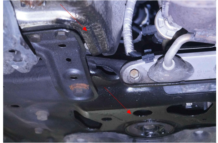
Bild 6: Technik, Motor, undicht, prüfen und Befund festlegen, Schaden- erweiterung möglich
