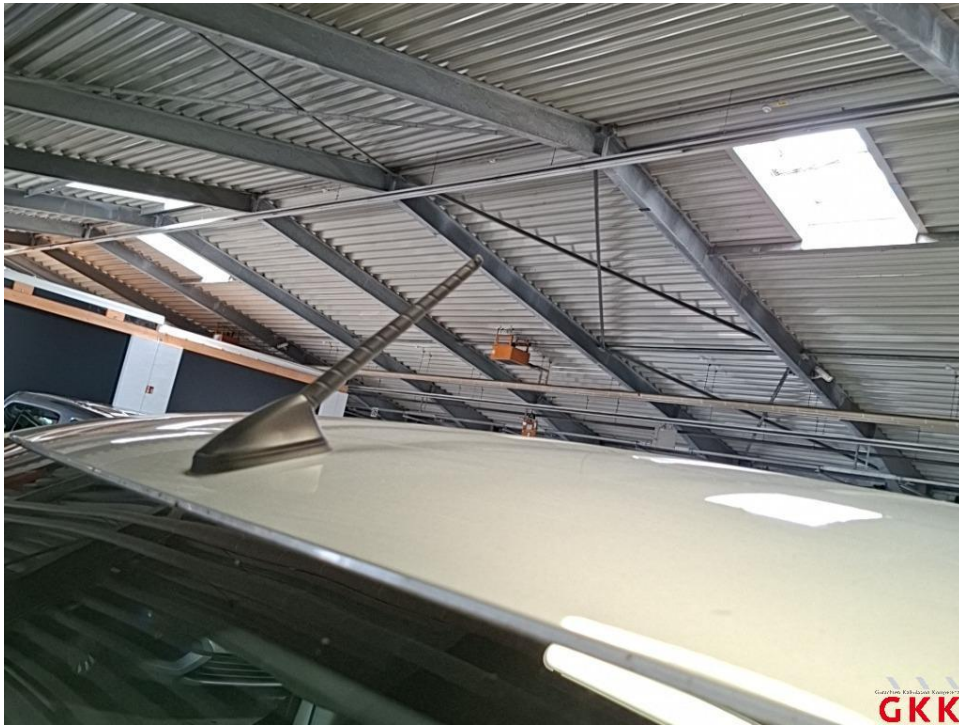
Bild 18 Antenne, Stab, beschädigt, ersetzen
