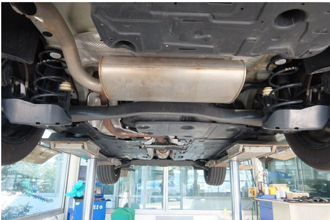
Bild 8 : Unterboden
