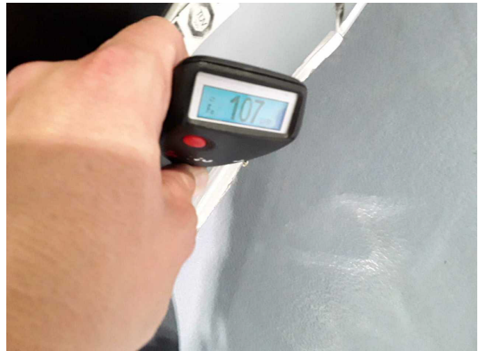
Schweller rechts: 107 \mu\text{m}
