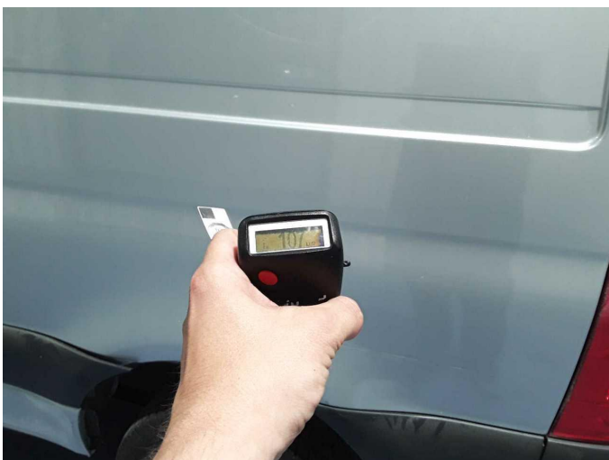
Seitenwand links: 107 \mu\text{m}
