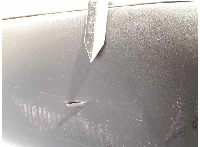
Beschädigung 32: Seitenwand links: Schutzleiste - gebrochen / gerissen - erneuern
