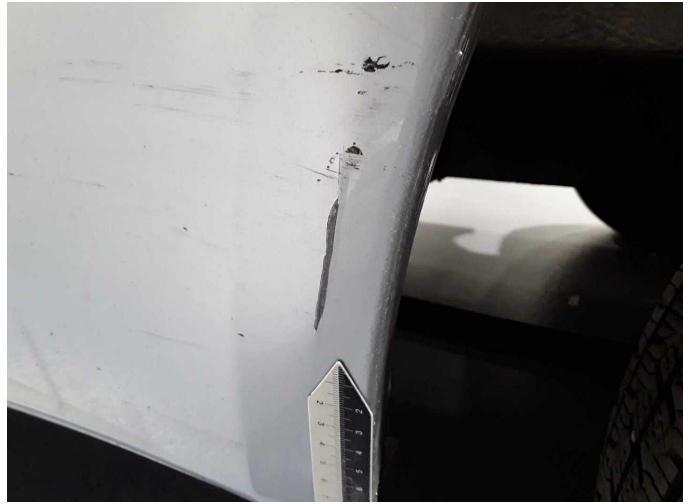
Beschädigung 30: Seitenwand links: Radlauf - verformt - instandsetzen/ lackieren (S3)
