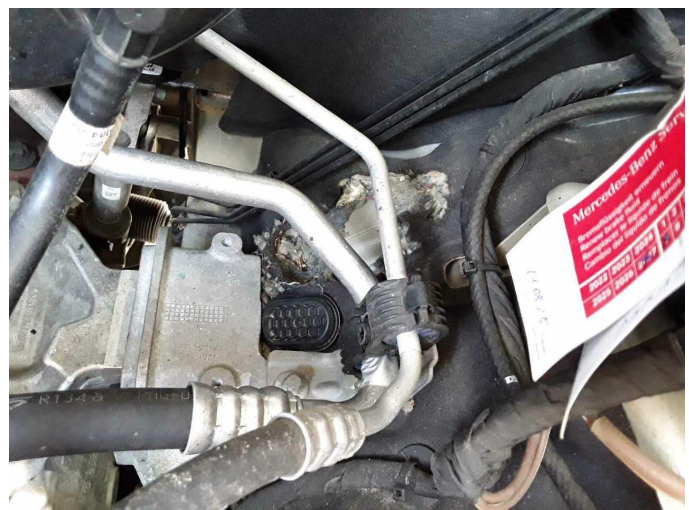
Beschädigung 2: Motor: Motorverkleidung - beschädigt - erneuern
