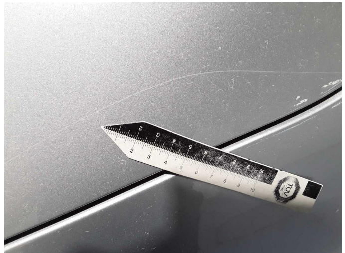
Beschädigung 36: Motorhaube: Motorhaube - verkratzt / verschuift - instandsetzen/lackieren (S3)
