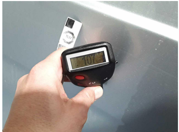
Seitenwand links: 107 \mu\text{m}
