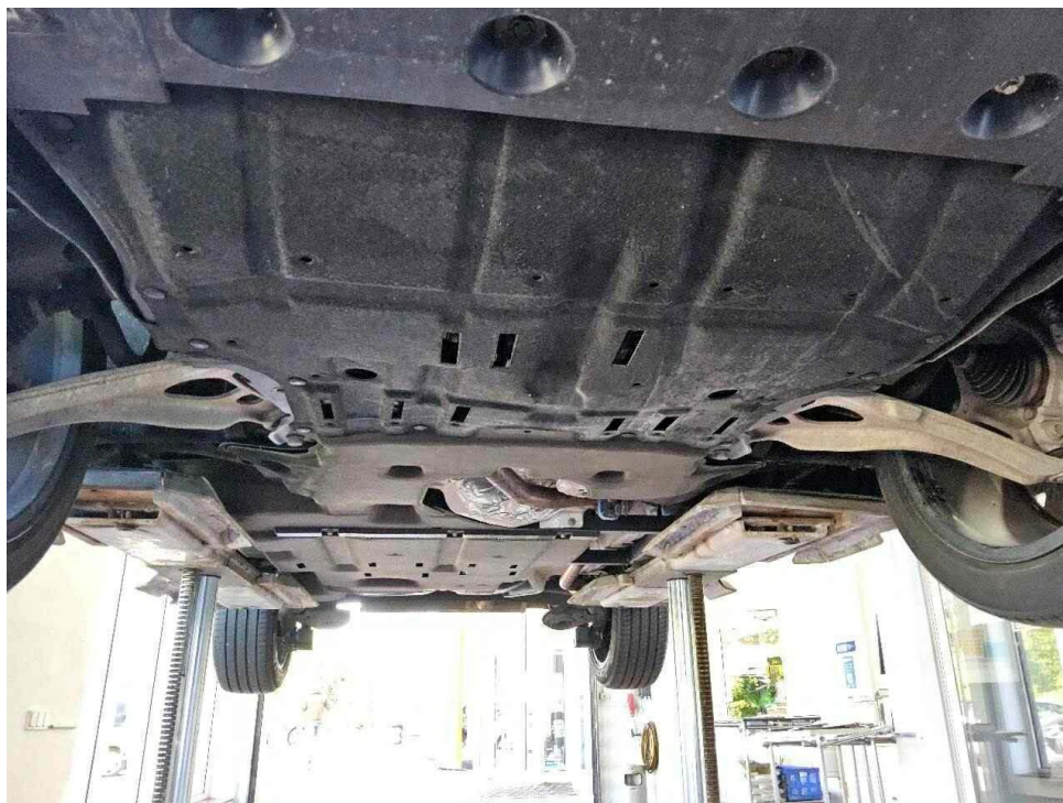
Bild 9 : Unterboden Schadenübersicht 8
