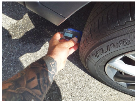
Set pneumatici principale / Anteriore Destro
