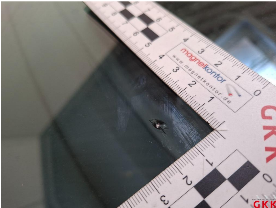
Bild 18. Frontscheibe, wärmedämmend mit Regensensor und Frontkamera, Steinschlag im Sichtfeld, ersetzen
