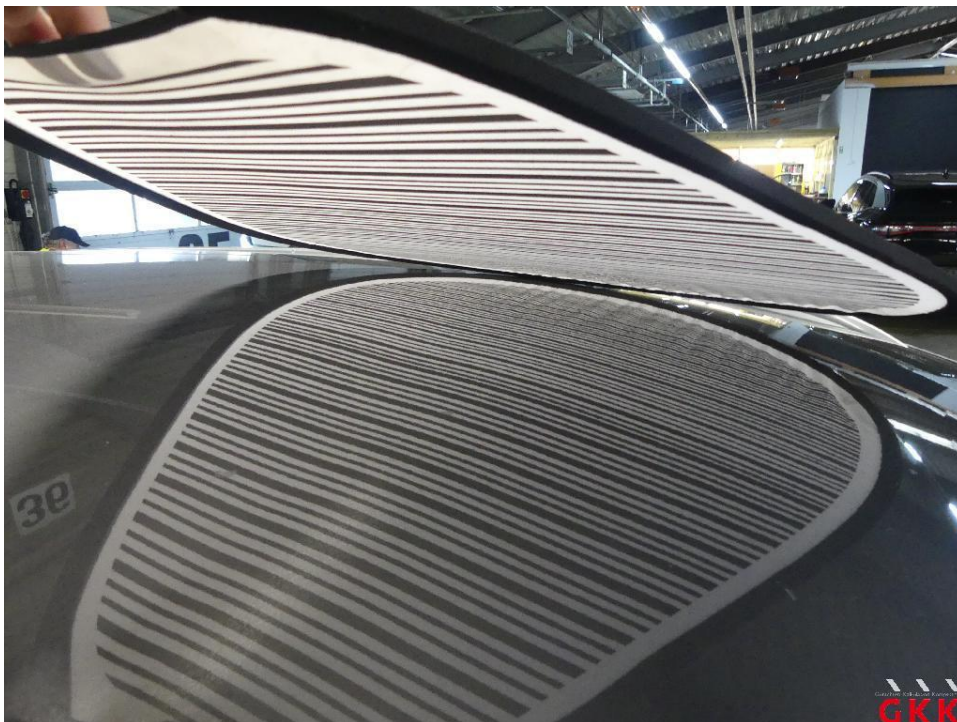
Bild 16 Fahrzeug, Hagelschaden, kalt drücken
