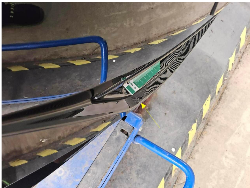
Bild 17 : Stoßfänger vorne, eingedellt, instandsetzen und lackieren mit Lackaufbau
