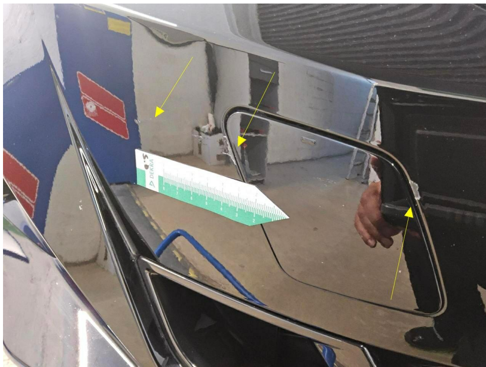
Bild 19 : Stoßfänger vorne, eingedellt, instandsetzen und lackieren mit Lackaufbau
