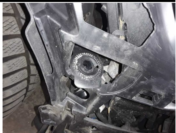
Beschädigung #11: Stossfänger vorn: Stossfänger mit Parktronic (Laut Ga.) - beschädigt - erneuern
