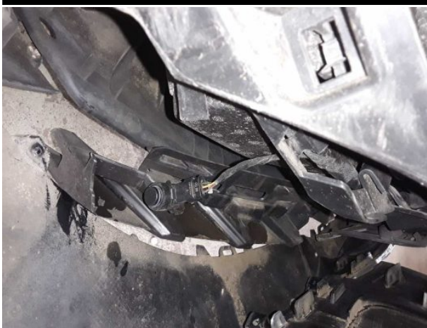
Beschädigung #11: Stossfänger vorn: Stossfänger mit Parktronic (Laut Ga.) - beschädigt - erneuern
