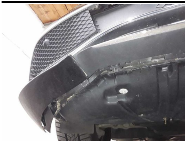
Beschädigung #4: Karosserie: Unterbodenverkleidung - gebrochen / gerissen - erneuern
