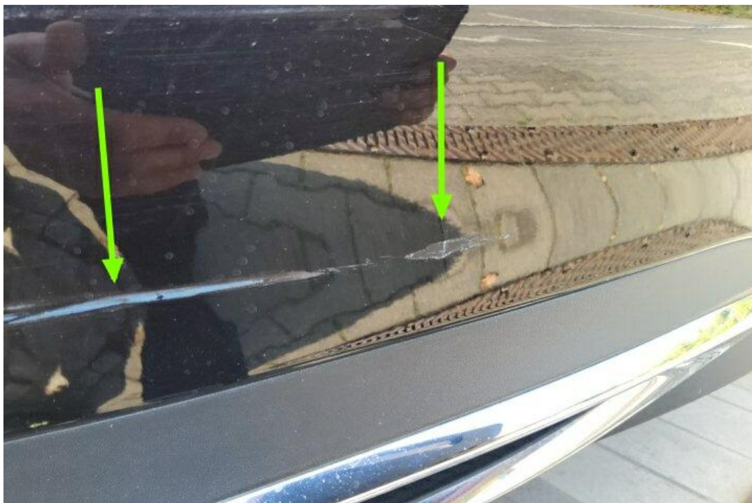
Bild 15 : Stoßfänger hinten Lackierung, zerkratzt, lackieren mit Lackaufbau
