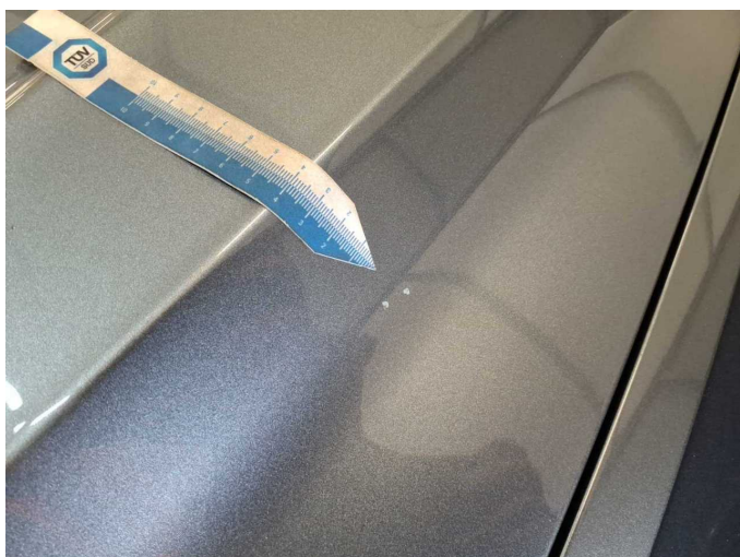
Damage 8: Bonnet: Bonnet (Steinschlag mit Korrosion) - Stone chips - Repair and paint
