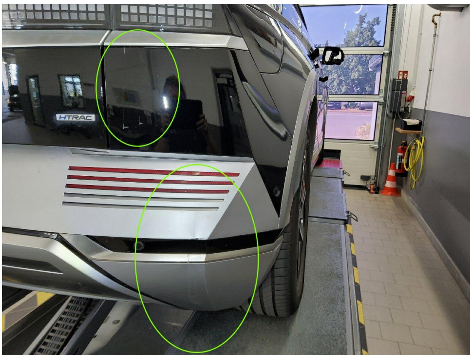
Bild 14 : Unfallschaden hinten rechts, Stoßfänger hinten deformiert
