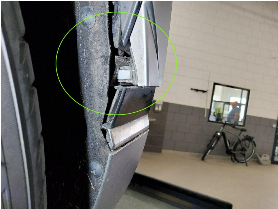
Bild 13 : Unfallschaden hinten links, Radhausschale, Stoßfänger hinten und Radlaufblende beschädigt
