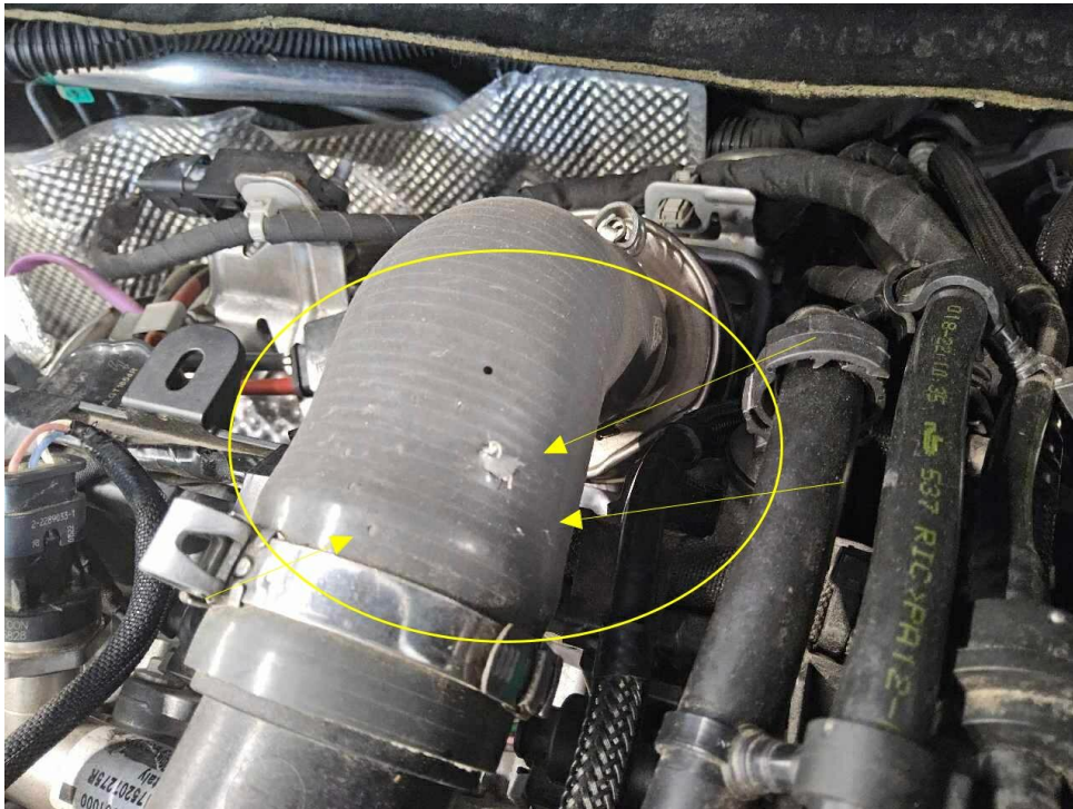
Bild 25 : Turboladerleitung eingerissen
