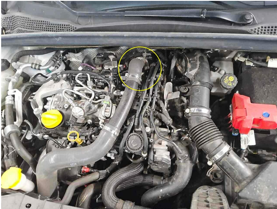
Bild 23 : Turboladerleitung eingerissen
