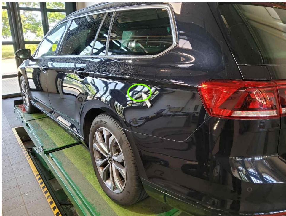
Bild 19 : Seitenwand hinten links, eingedellt
