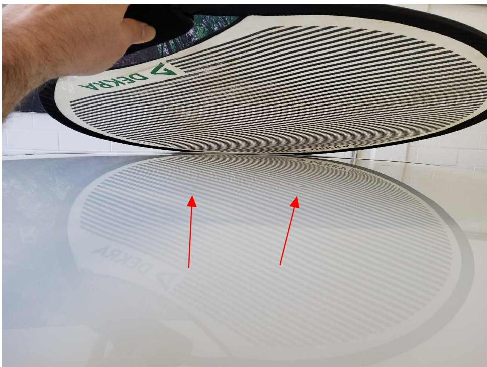
Bild 12 : Dach, mehrfach eingedellt
