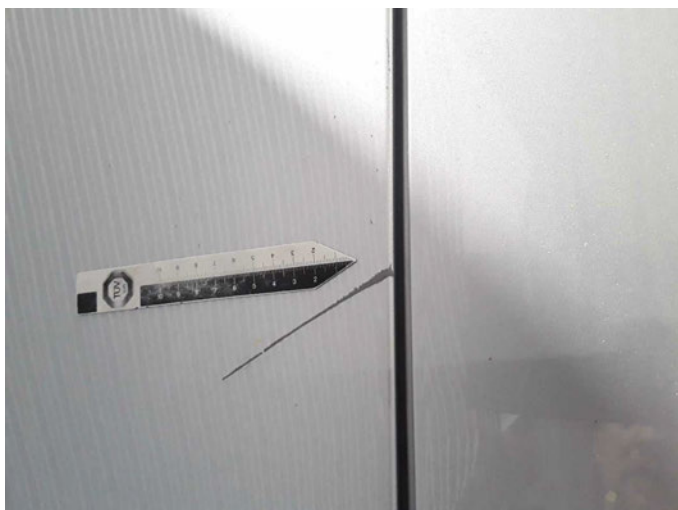
Beschädigung 23: Heckklappe/-tür: Hecktür links - nicht fachgerecht instandgesetzt - erneuern
