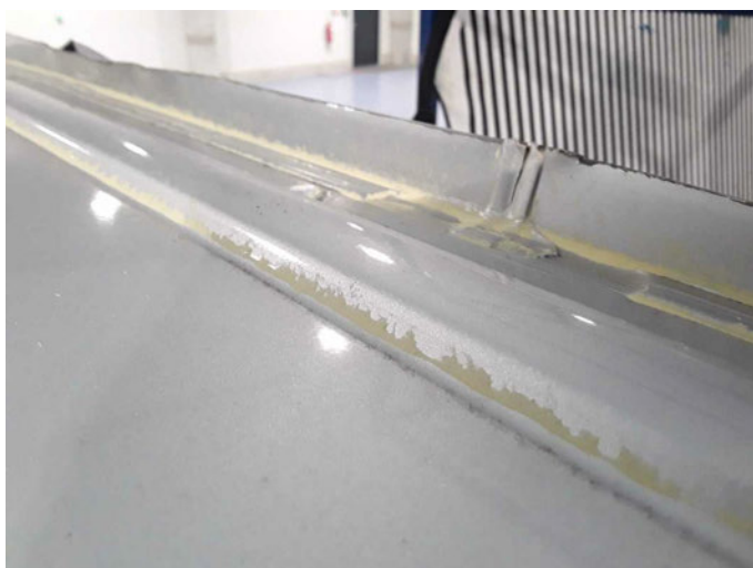
Beschädigung 44: Fahrzeugdach: Dachholm rechts - beschädigt - erneuern
