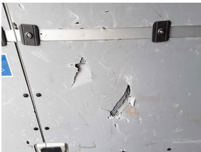
Beschädigung 4: Verkleidungen/Abdeckungen: Laderaumverkleidung links - beschädigt - erneuern
