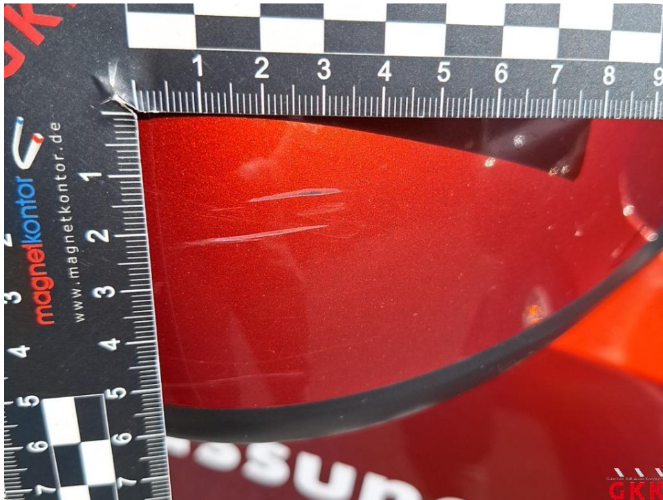
Bild 27 Spiegelgehäuse rechts, Kappe -lackiert-, verkratzt, lackieren
