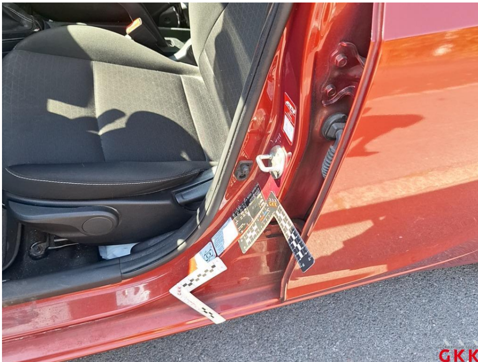
Bild 22 B- Säule links, beschädigt, instand setzen - lackieren
