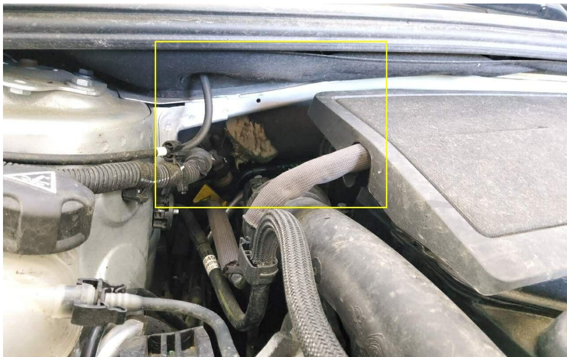
Bild 17 : Motorraum Dämmmatte Spritzwand Tierbiss
