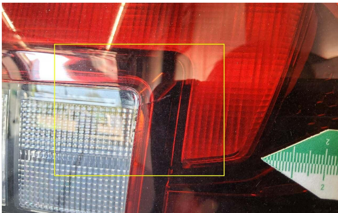
Bild 34 : Rückstrahler rechts außen gebrochen
