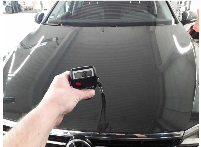
Bonnet: 330 \mu\text{m}
