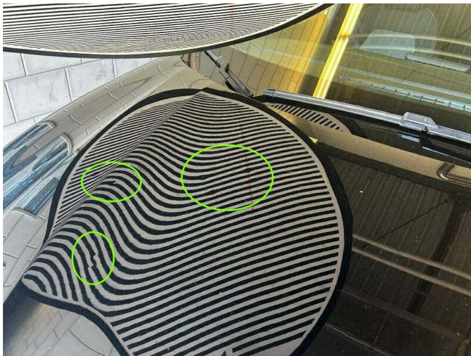
Bild 27 : Bestehender Hagelschaden
