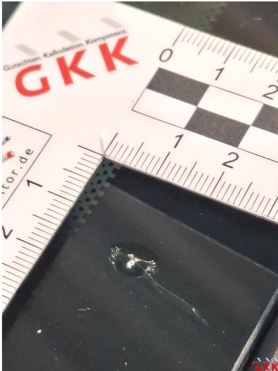
Bild 22 Frontscheibe, beschädigt, ersetzen
