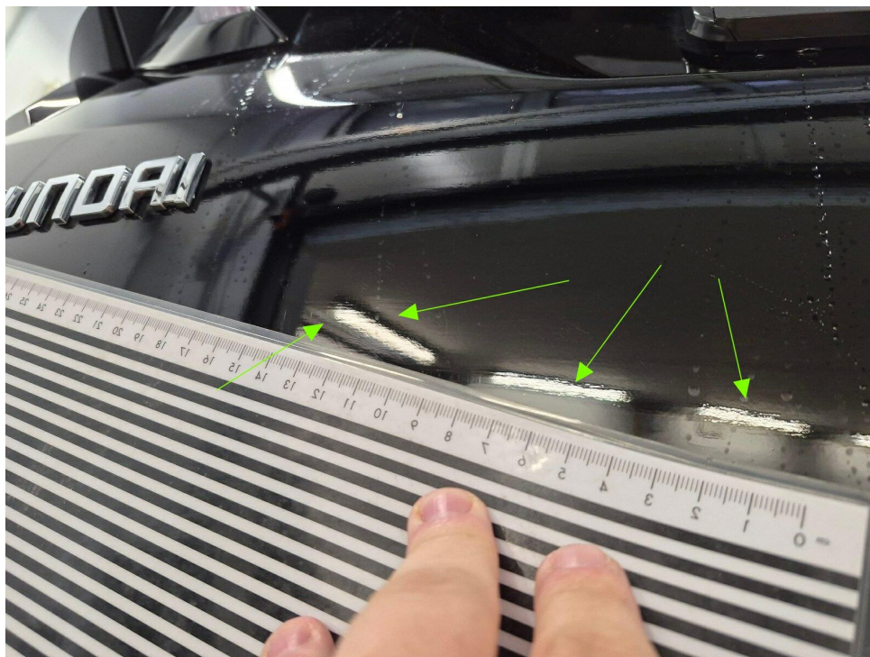
Bild 9 : Heckklappe Bearbeitungsspuren ersichtlich
