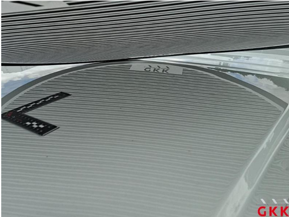
Bild 49. Dach, Hagelschaden, instand setzen
