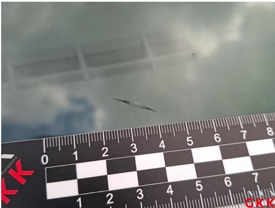
Bild 46. Frontscheibe, mit Regensensor, Steinschlag mit Rissbildung, ersetzen
