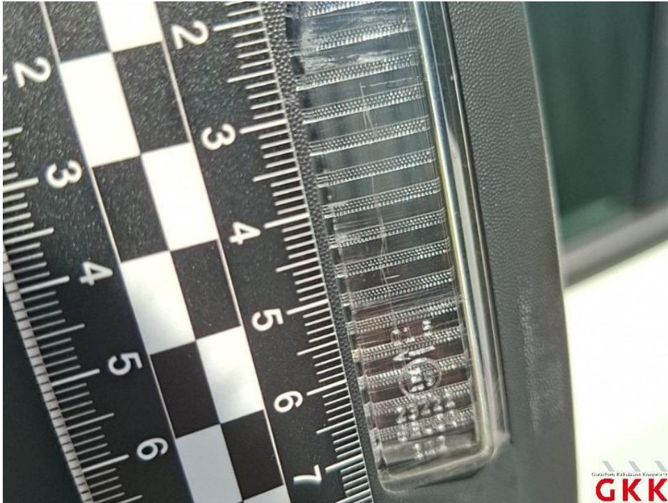
Bild 37. Spiegelgehäuse links, Blinker, verkratzt, ersetzen
