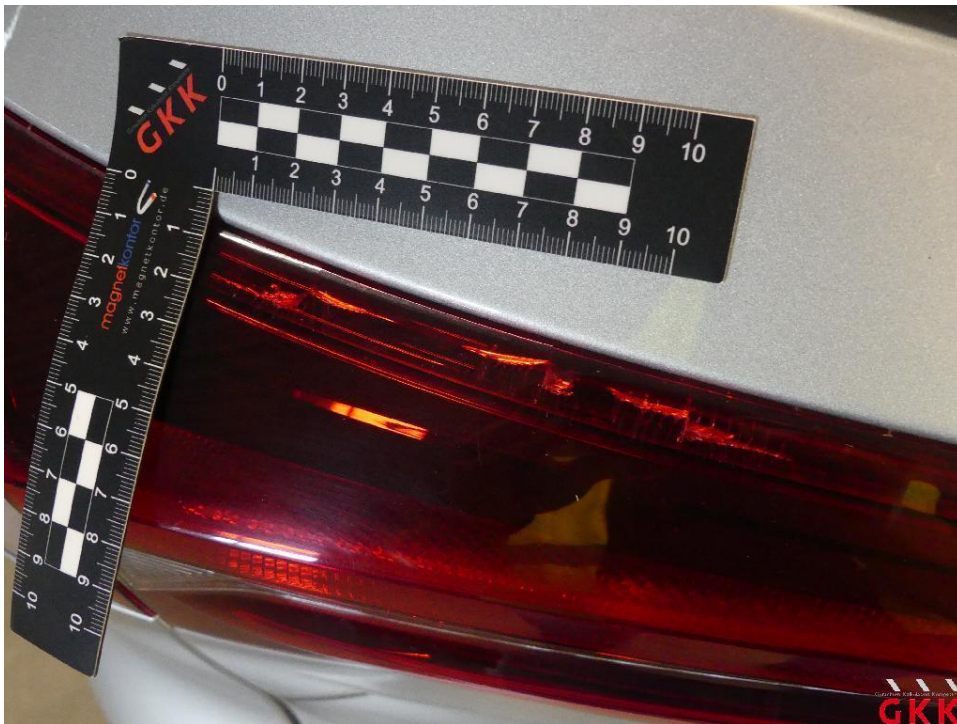
Bild 18 Rückleuchte links, innen, gerissen, ersetzen
