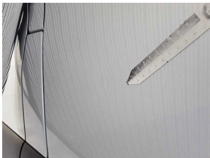
Beschädigung 26: Seitenwand links: Seitenwand - Delle / Lackschaden - sanft instandsetzen
