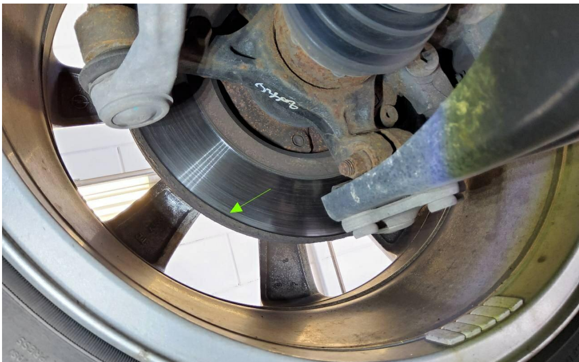
Bild 18 : T- Bremsscheiben Vorderachse eingelaufen
