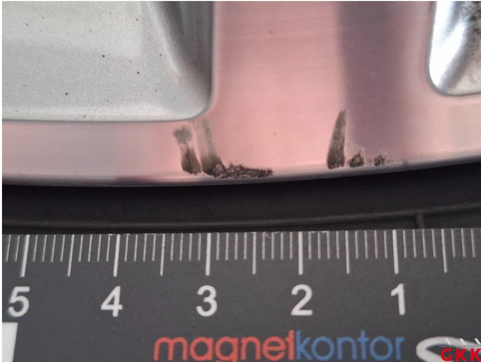
Bild 33. LM-Rad, vorne rechts, beschädigt, ersetzen
