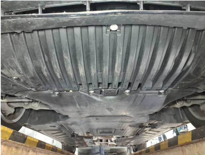
Abbildung 17: Unterboden
