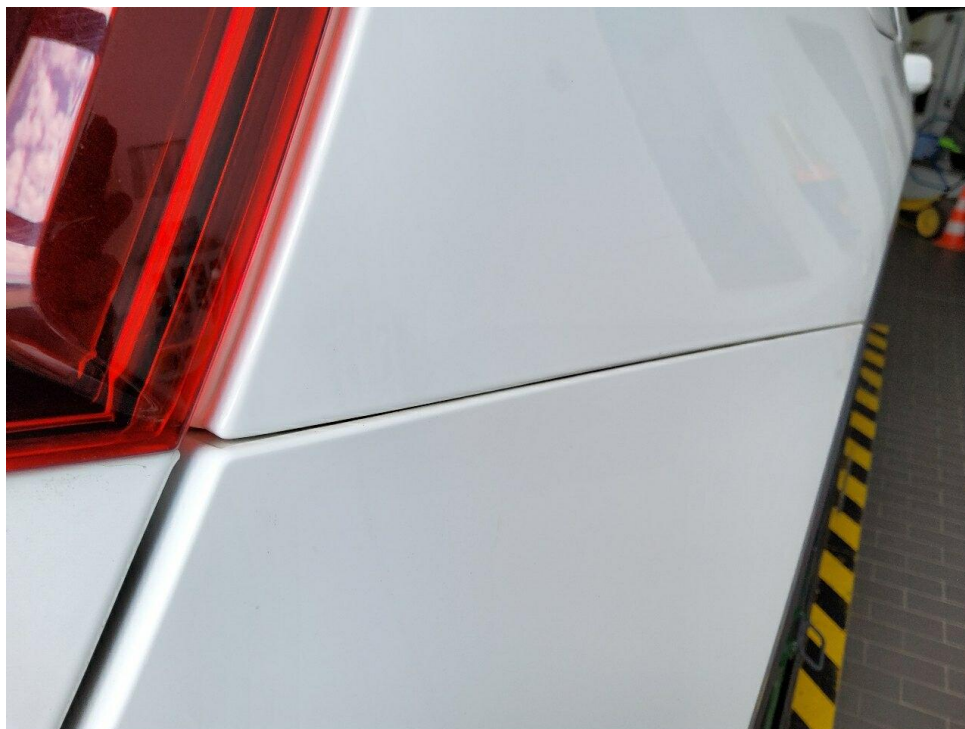
Bild 16 : Vergleich Spaltmaß Stoßfänger hinten rechts
