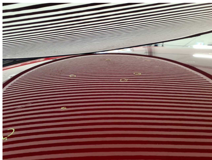
Damage 7: Roof: Roof (30 Dellen auf dem dach mit 2cm Durchmesser) - Damage by hail - Repair
