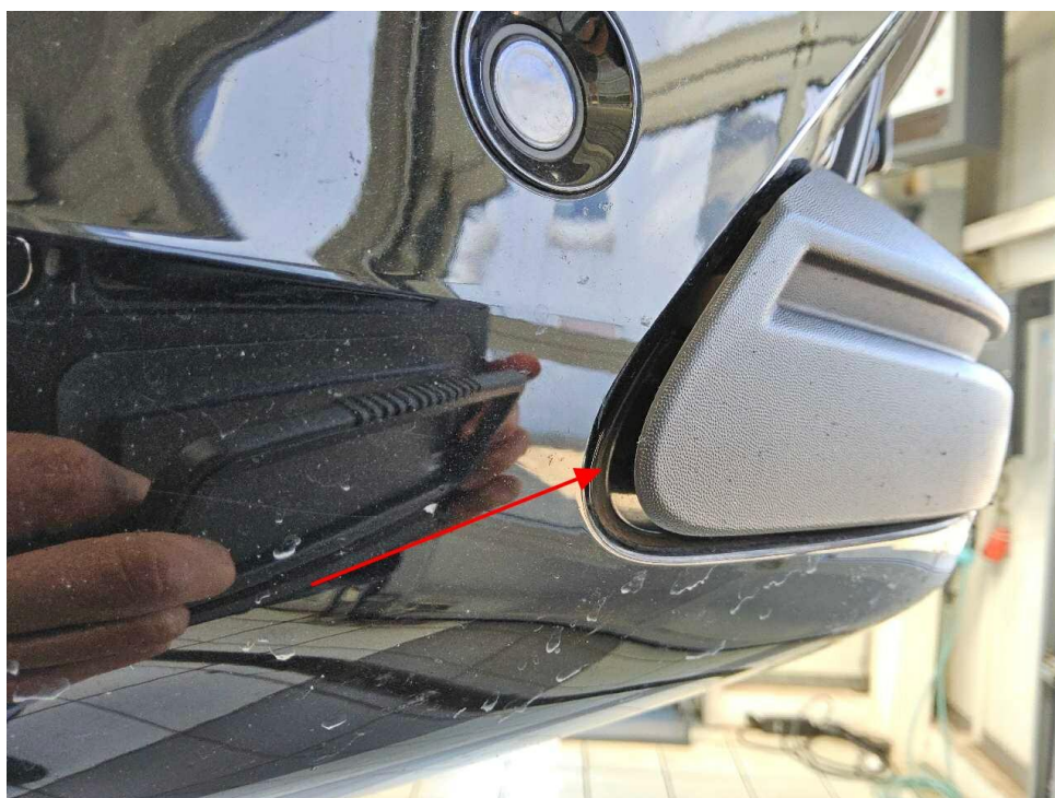
Bild 16 : Frontspoiler, verformt, erneuern
