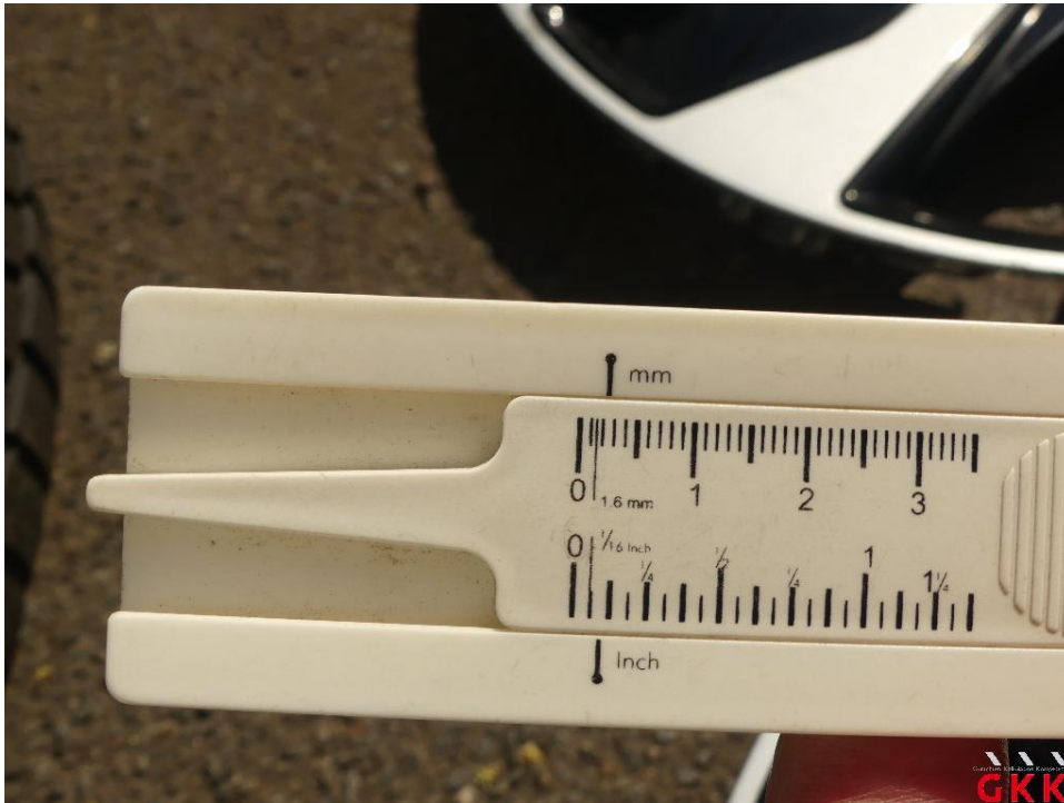
Bild 15. Reifen, 1 x beiliegend, Untermaß, ersetzen
