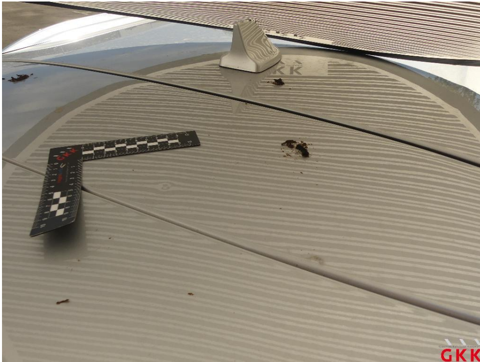
Bild 21. Heckklappe, bis 3 Dellen / Bauteil, kalt drücken
