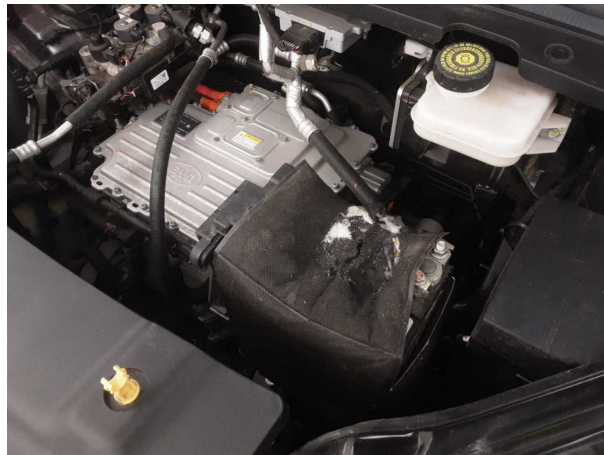
Beschädigung #1: elektrisches System: Batterieabdeckung - Marderschaden - erneuern
