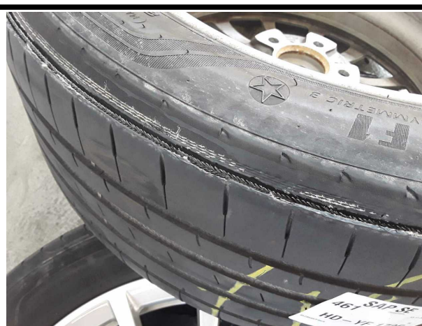
Beschädigung #5: 2.Radsatz: 2 Reifen - beschädigt - erneuern
