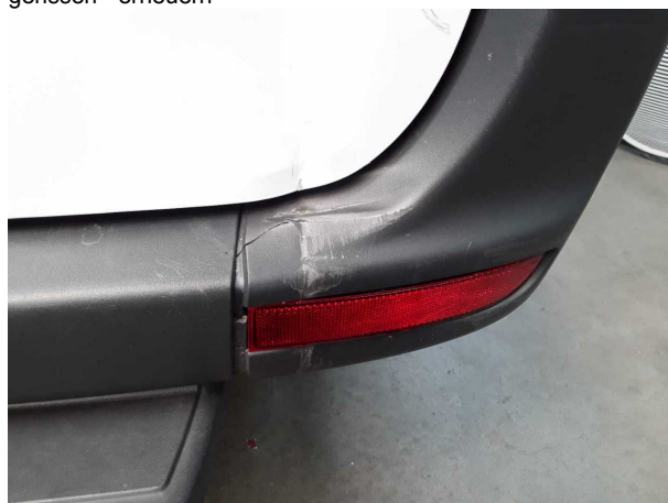
Beschädigung #4: Stossfänger hinten: Stossfänger hinten rechts (Mehrkosten können entstehen) - gebrochen / gerissen - erneuern
