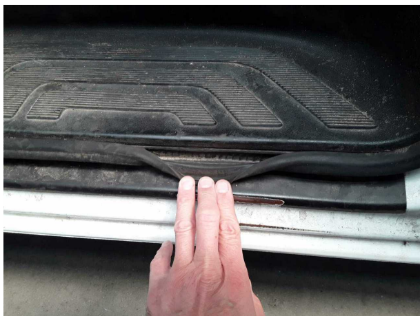
Beschädigung #1: Tür vorn links: Türdichtung - gebrochen / gerissen - erneuern
