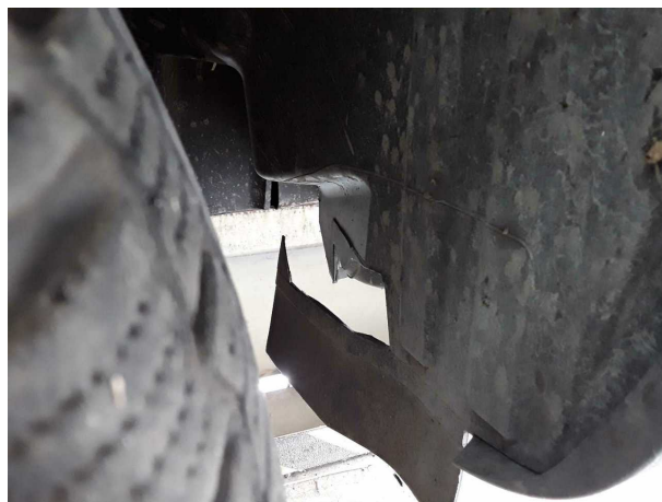
Beschädigung #2: Kotflügel rechts: Innenkotflügel - gebrochen / gerissen - erneuern
