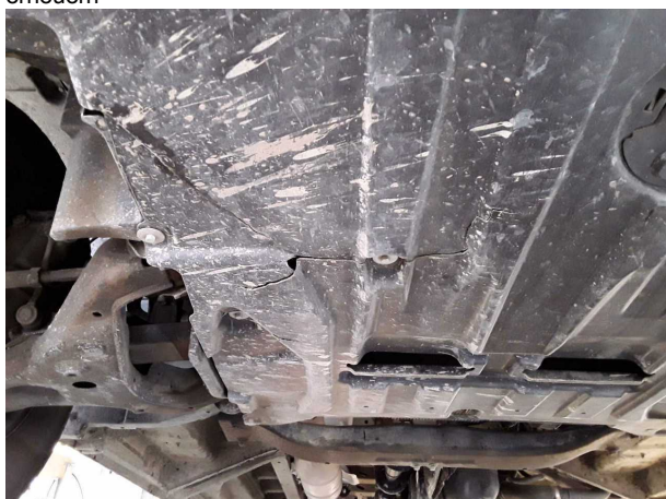
Beschädigung #3: Motor: Motorverkleidung unten - gebrochen / gerissen - erneuern
