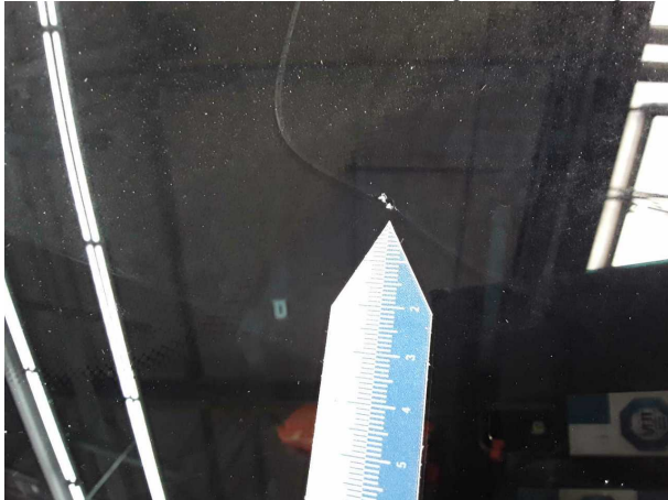
Beschädigung #10: Verglasung: Frontscheibe mit Spurhalteassistent - Steinschlag - erneuern
