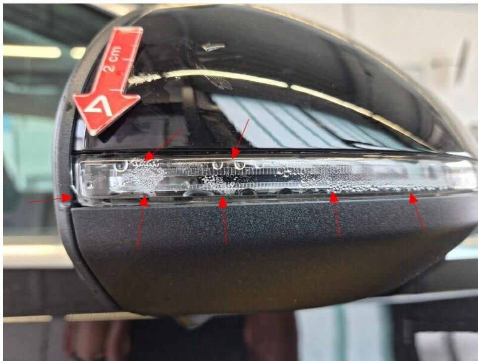
Bild 17 : Tür vorn rechts Aussenspiegel Zusatzblinkleuchte gebrochen mit Feuchtigkeitseintritt
