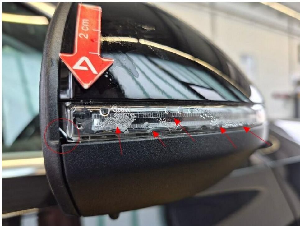
Bild 16 : Tür vorn rechts Aussenspiegel Zusatzblinkleuchte gebrochen mit Feuchtigkeitseintritt
